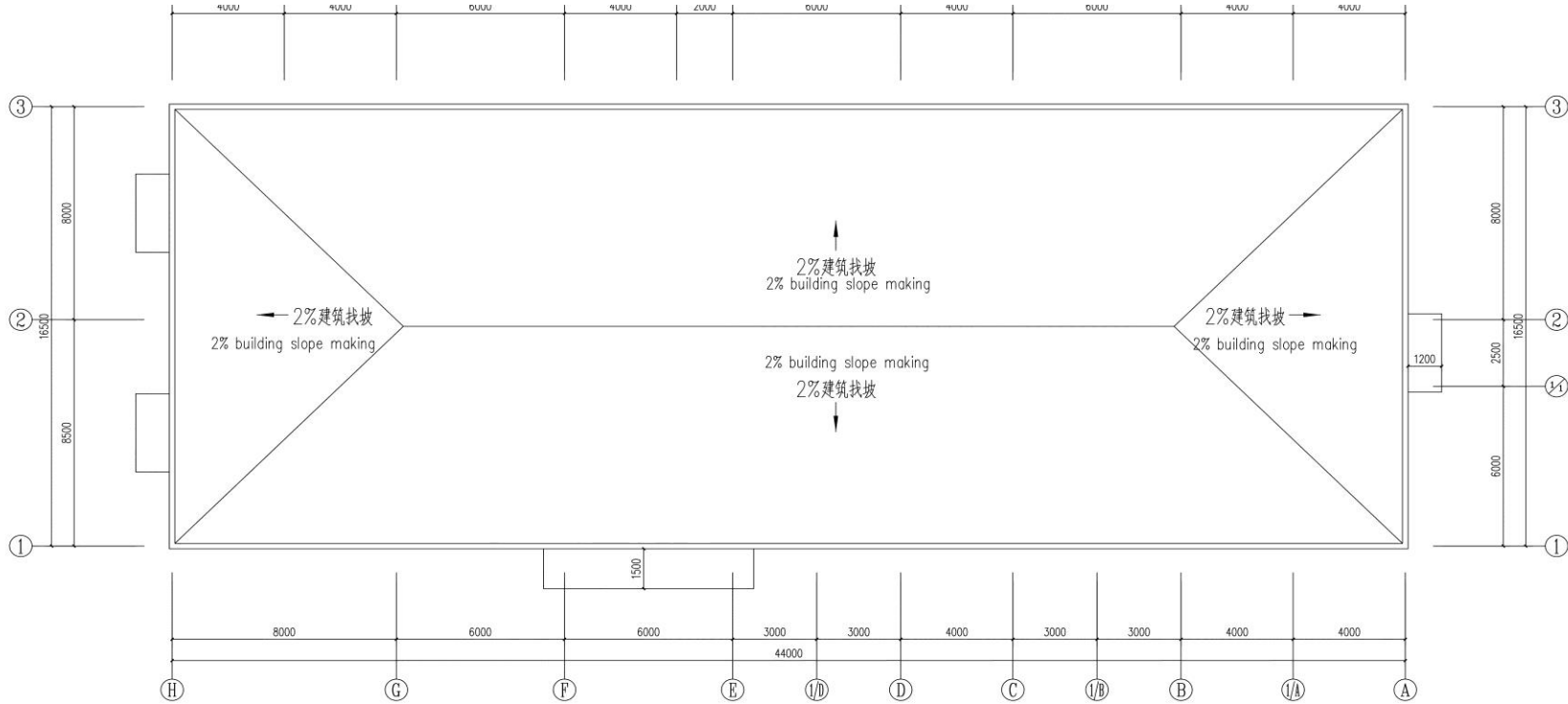
屋顶平面图 Roof plan 1:100
