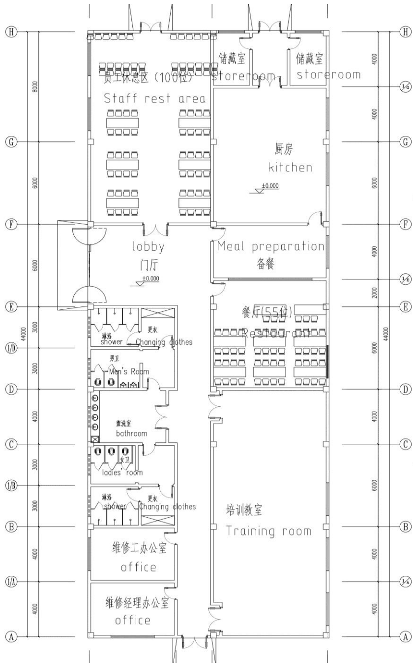
一层平面图
