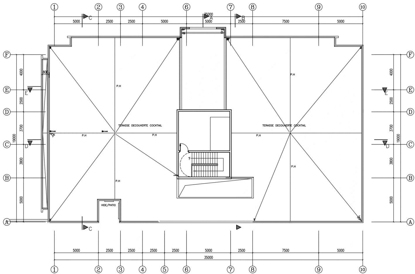
屋顶层平面 1:100
