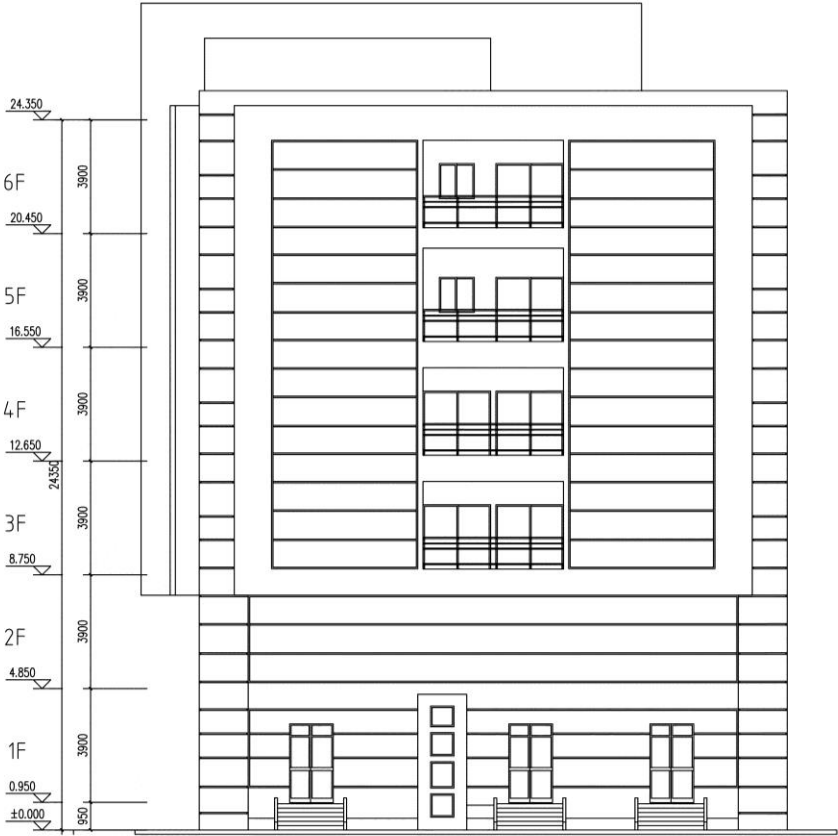
West elevation 1:100 西立面 1:100
