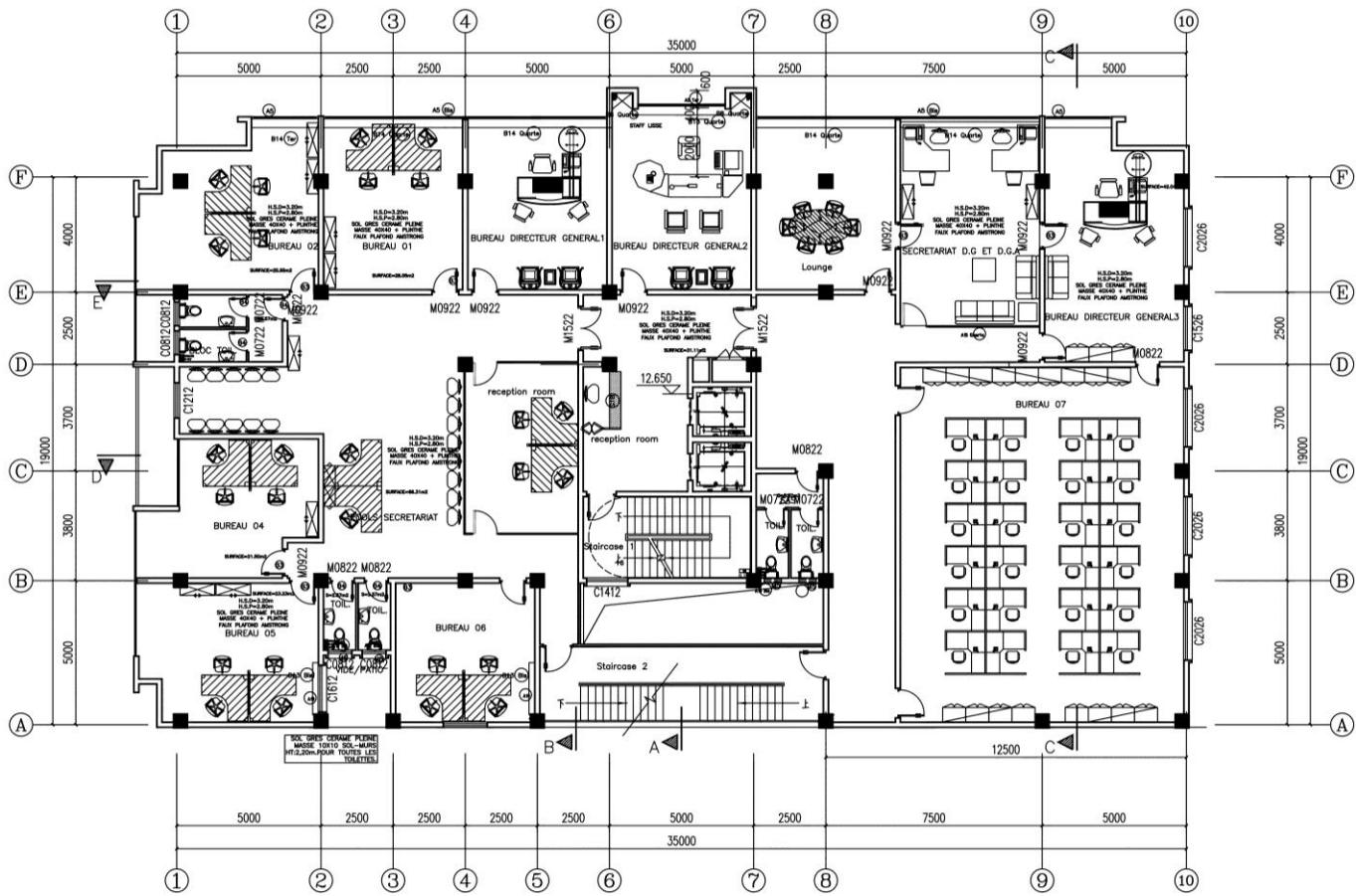
四层平面 1:100
