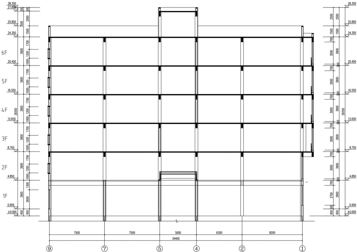
Section view 1:100 剖面图
