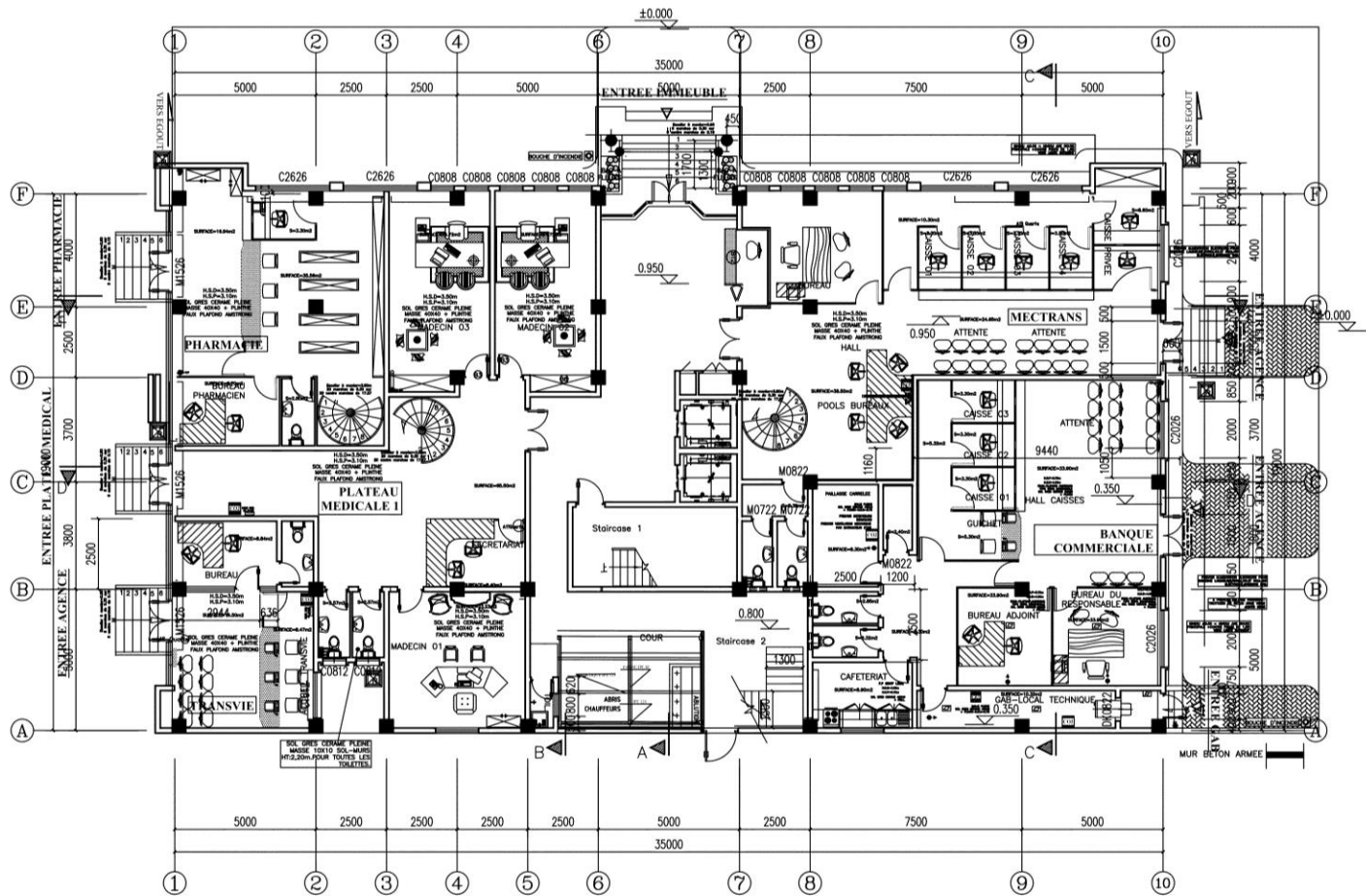
一层平面 1:100
