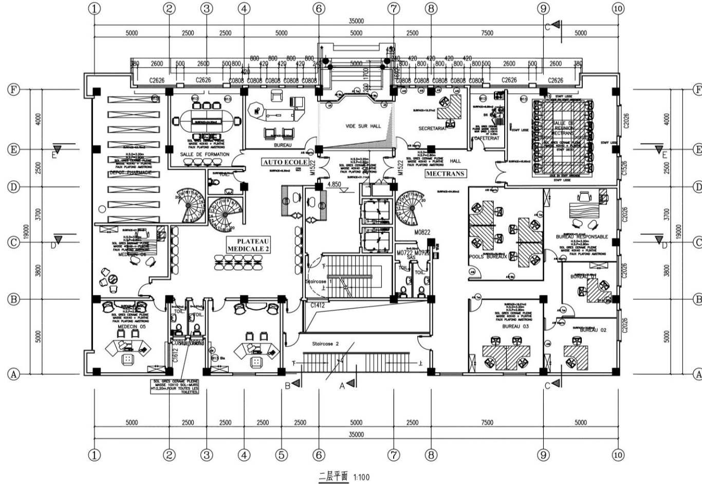
二层平面 1:100
