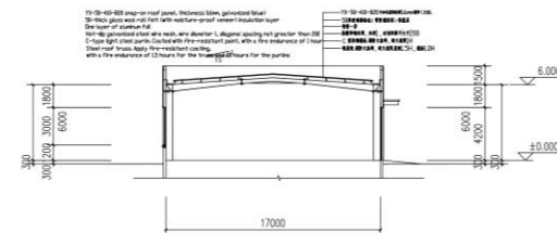
1-1剖面图
