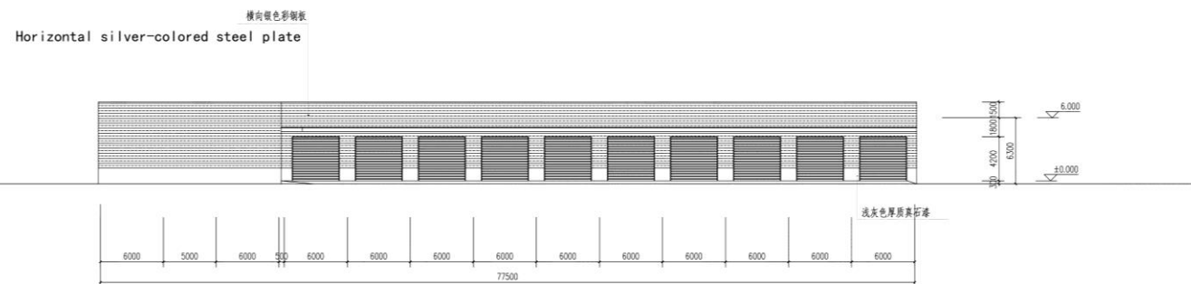
东立面图
