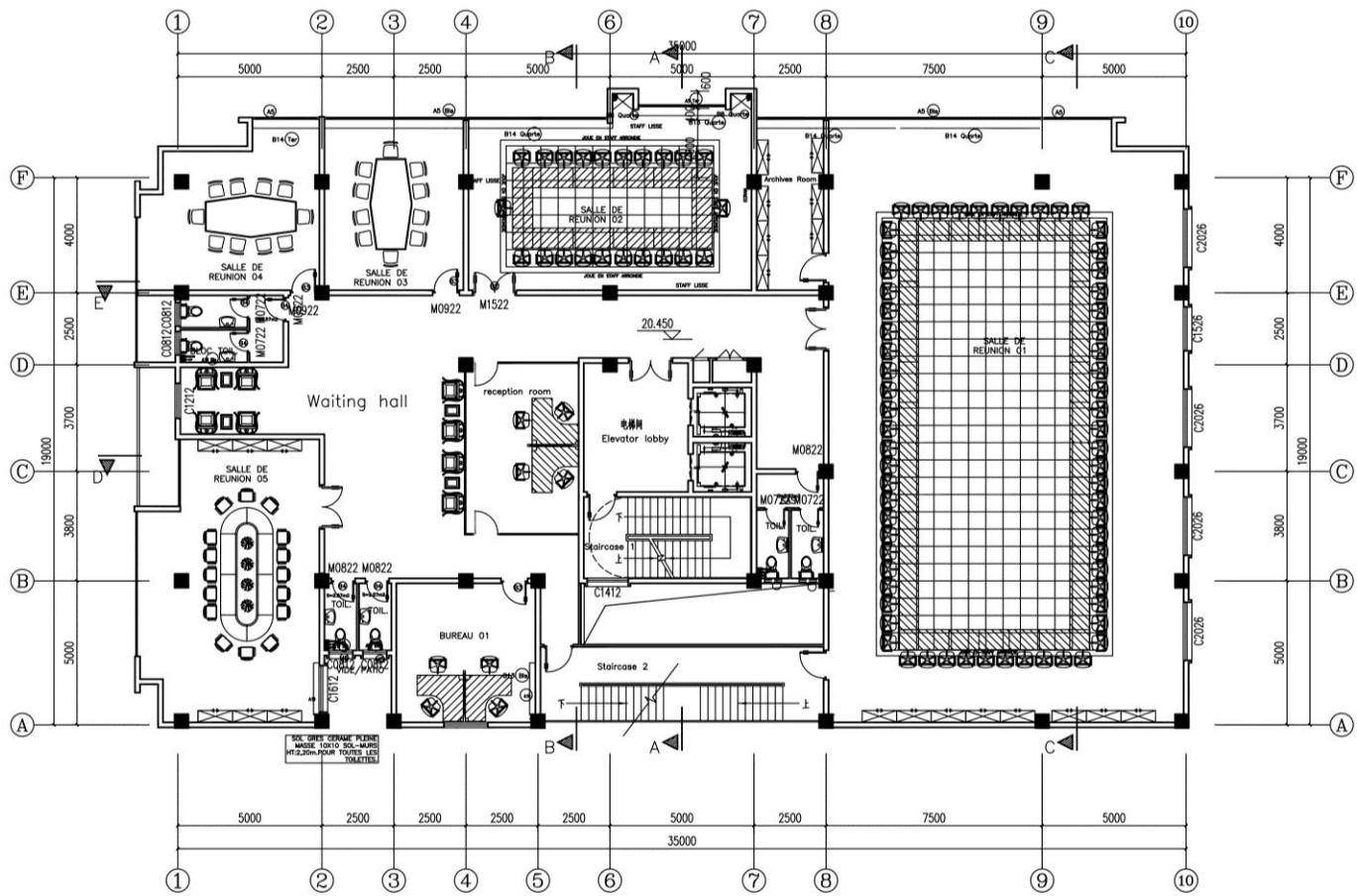
六层平面 1:100
